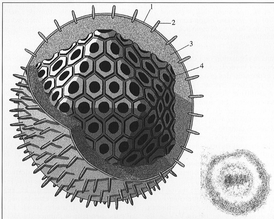
Figure 1. Schéma de la structure du VZV. La particule virale a un diamètre d'environ 200 nm et est entourée d'une enveloppe lipidique (1) dans laquelle sont ancrées plusieurs glycoprotéines (2) appelées gE, gB, gC, gH, et gI. Sous l'enveloppe virale, se trouve un tégument protéique (3) qui renferme plusieurs protéines régulatrices comme, par exemple, IE4, IE62 et IE63. La capsidie du VZV (4) est icosaédrique et composée de 162 capsomères hexagonaux. À l'intérieur de la capsidie est enfermé l'ADN en double chaîne qui comprend 124 884 paires de bases. L'ADN est composé de deux segments uniques: U L (104 836 bp) et U S (5 232 bp). Ceux-ci sont entourés d'éléments répétés: TR L et IR L (88,5 pb) et TR S et IR S (7 319,5 pb). L'ADN viral comprend 71 cadres de lecture ouverts dont trois sont en deux copies (ORF 62, 63 et 64). En encart, photographie en microscopie électronique d'une particule virale (grossissement x100 000).
